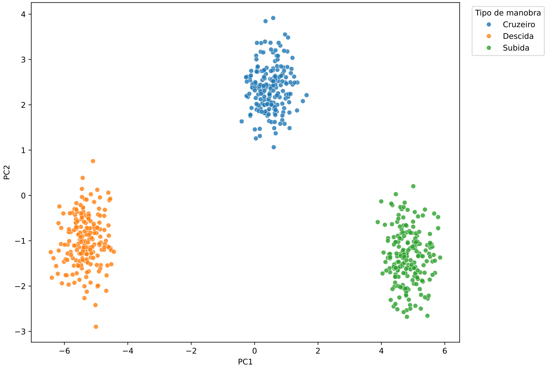
Projeção PCA 2D — PC1 vs. PC2
